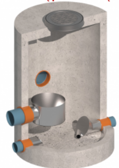
Regulator stożkowy z komorą przelewową
